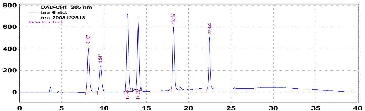
兒茶素標準品HPLC圖
