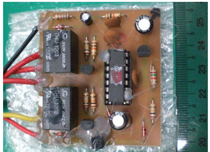
單鍵啟閉開關控制器實體圖
