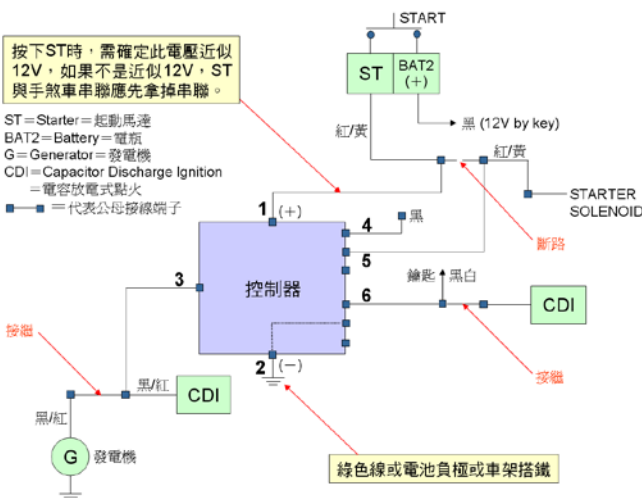
單鍵啟閉開關控制器線路圖
