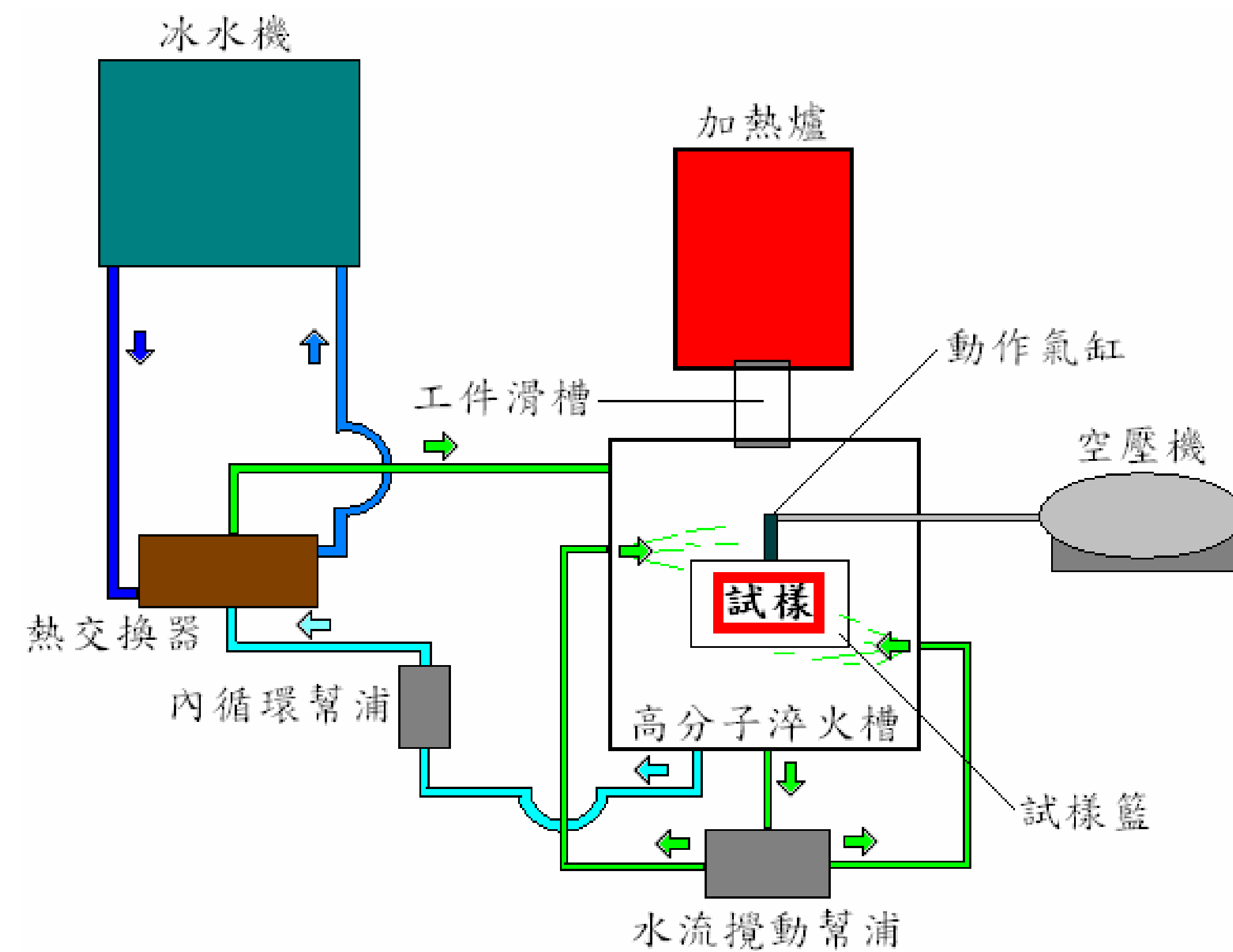
(a) 實驗系統主要設備示意圖
