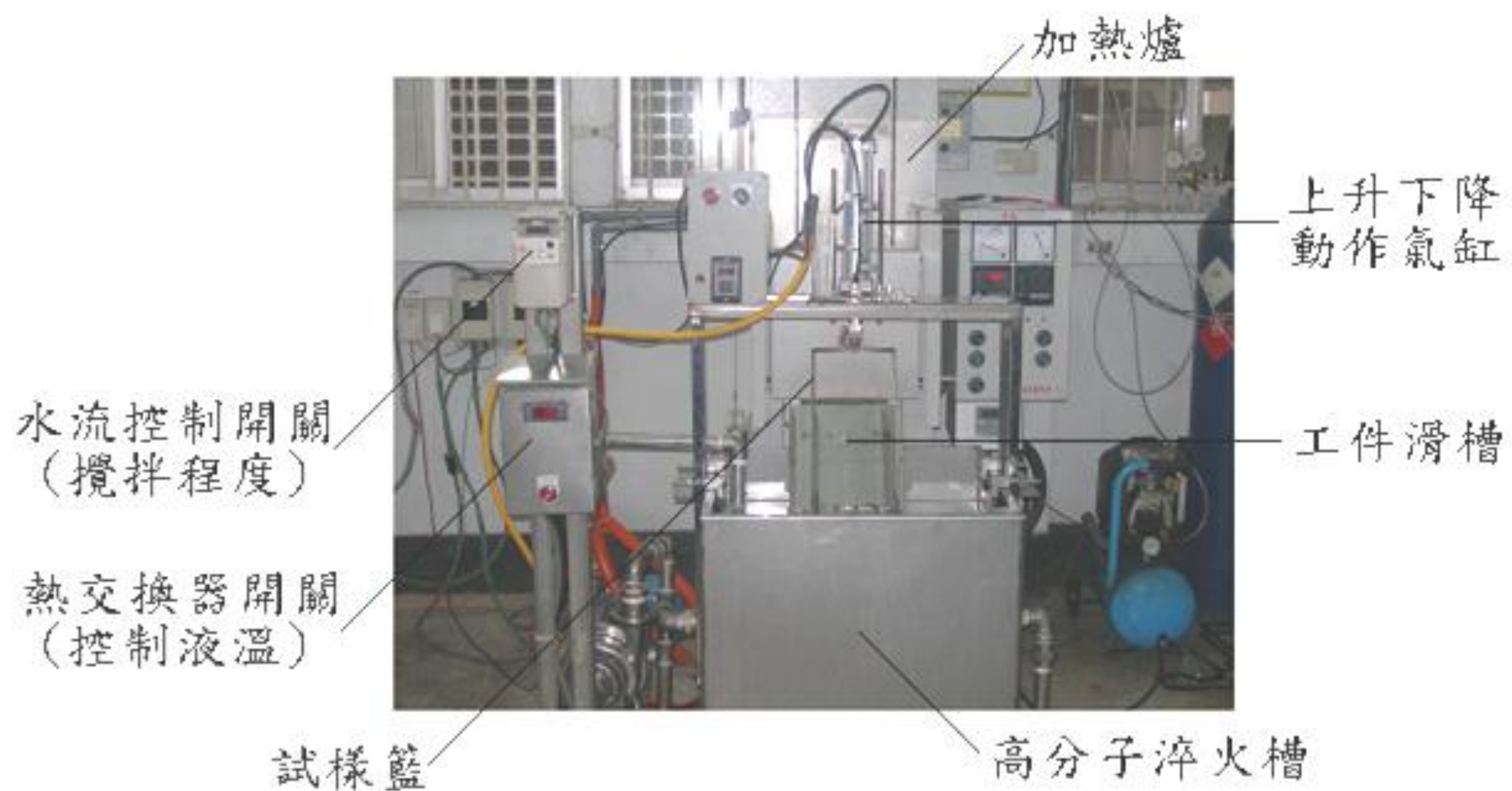
(b) 實驗設備照片
